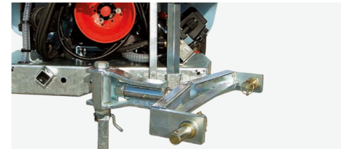
Timone articolato con cuscinetti / Tracker drawbar with bearings / Attelage articulé avec roulements / Gelenkdeichsel mit Lager / Tiro articulado con cojinetes
