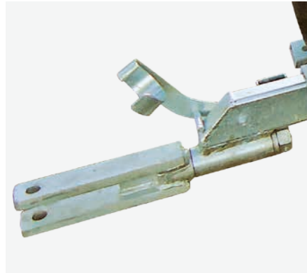
Timone a forcella / Clevis drawbar / Attelage a chappe / Deichsel mit Anhängegabel / Tiro de forquilla
