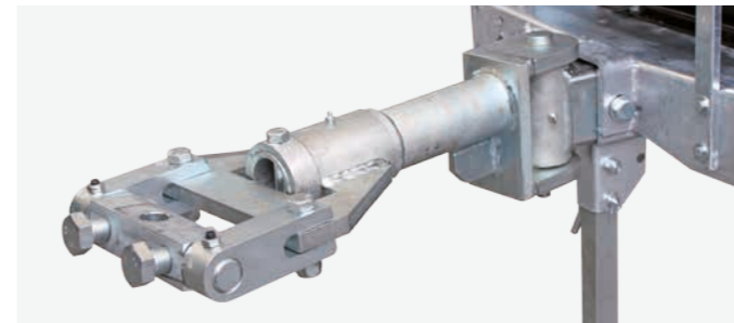
Timone sterzante con cuscinetti tipo Germania / Tracker drawbar with bearings "German type" / Attelage articulé monté sur roulement modèle Germania / Lenkdeichseln mit Lager Germania Modell / Tiro articulado con cojinetes tipo Alemania
