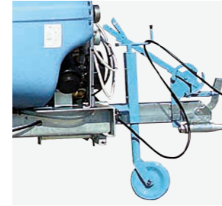
Ruotino appoggio / Tournig wheel / Support Béquille jockey / Stützrad / Rueda de apoyo
