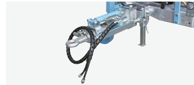
Timone sterzante omologato stradale/bloccaggio idraulico (option) / Tracker drawbar for road approval/hydraulic lock (optional) / Attelage articulé routier/option blocage hydraulique / Lenkdeichsel für verkehrszugelassene Maschinen (hydraulische Blockierung-Option) / Tiro articulado para homologación de carretera/bloqueo hidráulico (opcional)
